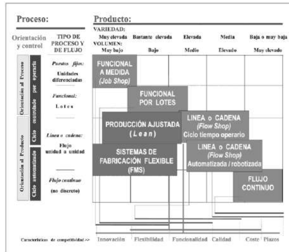
Figura 2. Diseño de procesos y plantas de producción flexible. Fuente: (Cuatrecasas, 2009).
